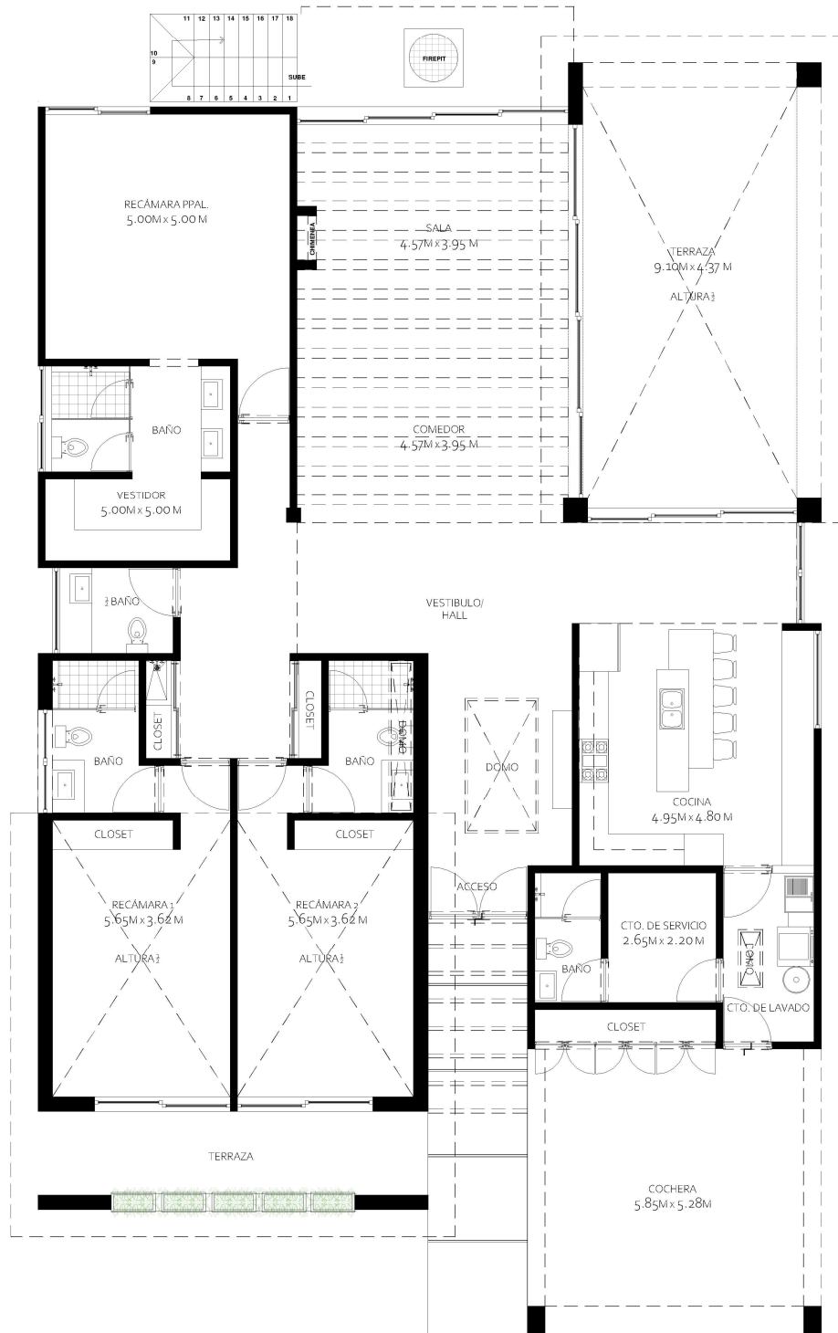
PLANTA BAJA REMEDIOS - CASA SOL
